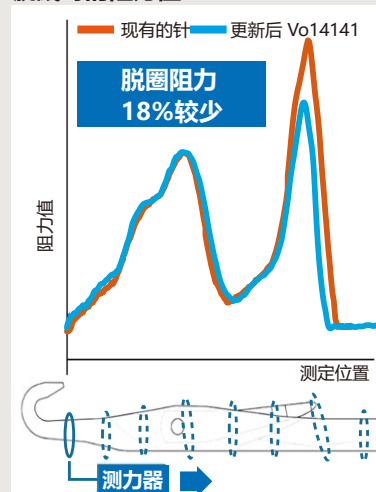
脱圈时的阻力值
