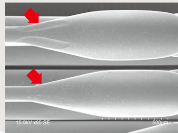
同样使用期间的针舌磨损状态
